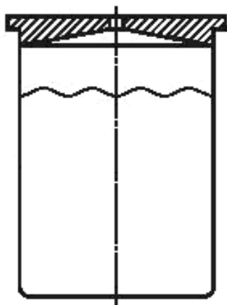
Рисунок 1 — Металлический пикнометр
